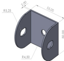
Roof Profiles upper falnges Çatı Profili Üst Flanşı 50 x 55 x 2 mm
