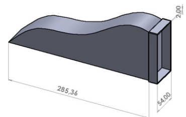
Roof Profiles Cover Cups Çatı Profili Tıpası 285 x 54 x 3 mm
