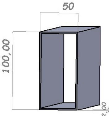
Roof Profiles / Çatı Profili 100X50X2
