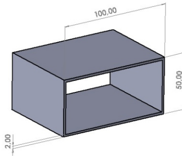
Wall Support Profile Duvar Bağlantı Profili 100X50X2 mm
