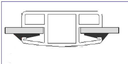
Roof Profiles / Çatı Profili 60 x 20,5 x 2mm
