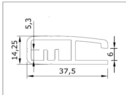
Sheet Cup Front Profiles Çatı levhası ön Profili
