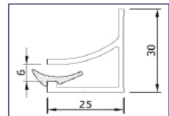
Sheet Cup Rear Profiles Çatı levhası arka Profili
