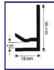
Front Profile Ön Profil
