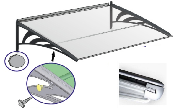
Arm Front Cap Kol Ön Kapağı
